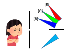
等色関数
