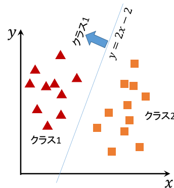
この (w_0, w_1, w_2) はよさそう パーセプトロンは特徴空間を超平面で分割する手法
